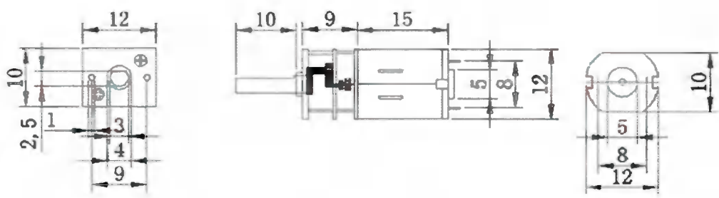
图 2 电动机尺寸参数（供参考，单位：mm）
